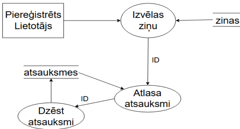
4.6. att. Datu plūsmu diagramma savas atsauksmes dzēšanai
