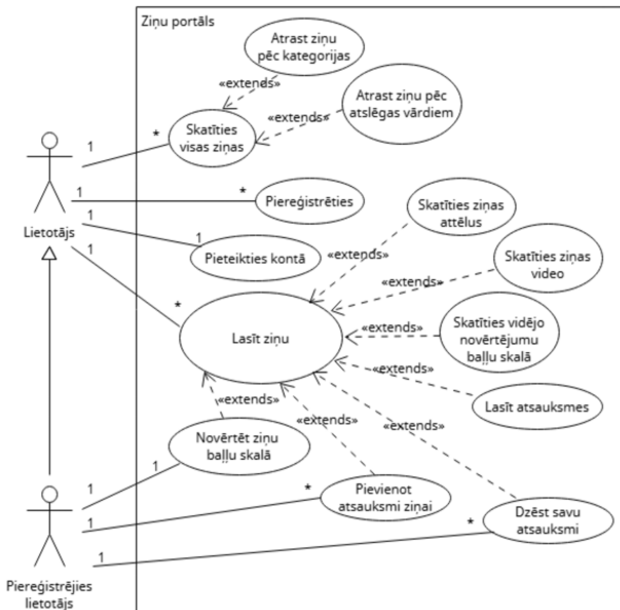
2.1. att. Lietojumu gadījumu diagrammas pirmā daļa
